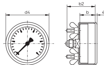
Typ R16.H.4.N... *) Dreikantfrontring triangular bezel collerette avant triangulaire
