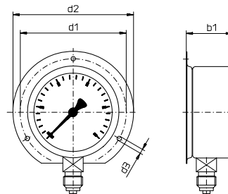
Typ R16.U.3.N... Rand hinten surface mounting flange rebord arrière
