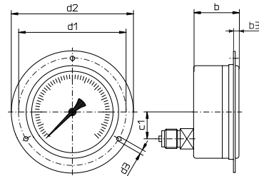
Typ R14.H.2.N... Rand vorne panel mounting flange collerette avant
