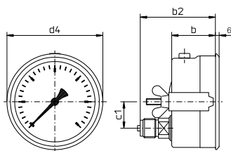
Typ R11.H.4.N... *) Dreikantfrontring triangular bezel collerette avant triangulaire
