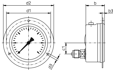
Typ R11.H.2.N... Rand vorne panel mounting flange collerette avant
