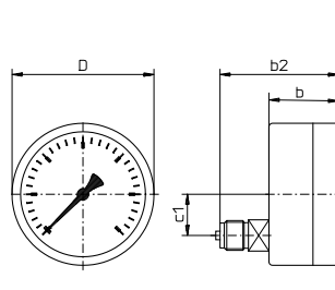
Typ R10.H.1.N... Anschluss hinten back pressure entry raccord arrière
