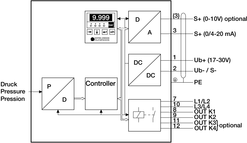
Anschlussbelegung Wiring details raccordement
