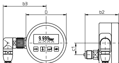
Typ ME25.H.1.N... Anschluss hinten back pressure entry raccord arrière
