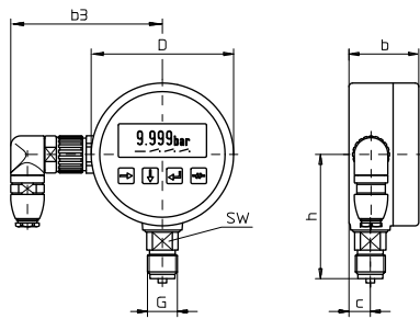
Typ ME25.U.1.N... Anschluss unten bottom pressure entry raccord en bas
