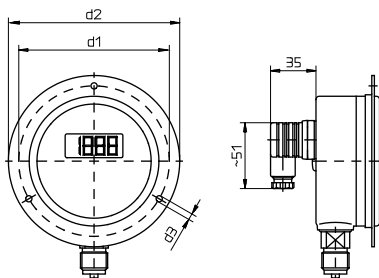
Typ ME20.U.2.N... Rand vorne panel mounting flange colletette avant
