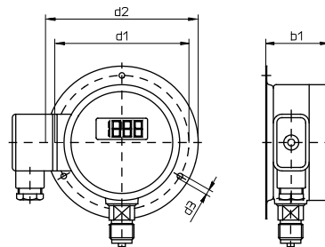
Typ ME20.U.3.N... Rand hinten surface mounting flange rebord arrière
