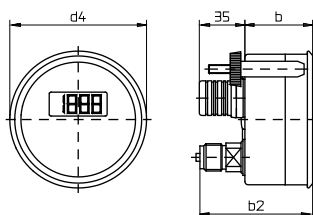
Typ ME20.H.4.N...*) Dreikantfrontring triangular bezel colletette avant triangulaire
