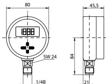
Typ ME20.U.1.N... Anschluss unten bottom pressure entry raccord en bas
