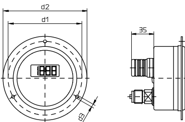
Typ ME20.H.2.N... Rand vorne panel mounting flange colletette avant
