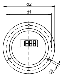
Typ ME10.H.2.N... Rand vorne panel mounting flange collerette avant
