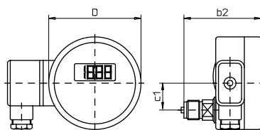
Typ ME10.H.1.N... Anschluss hinten back pressure entry raccord arrière
