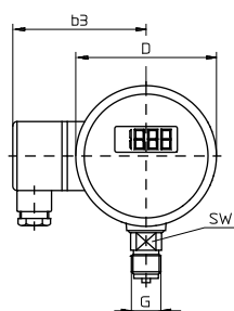
Typ ME10.U.1.N... Anschluss unten bottom pressure entry raccord en bas
