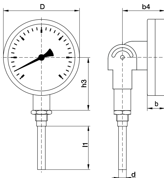
Typ B20.S.7.N... Anschluss schwenkbar mit Halsrohr (>300°C) Swiveling connection with neck extension (>300°C) Raccord orientable avec prolongement (>300°C)
