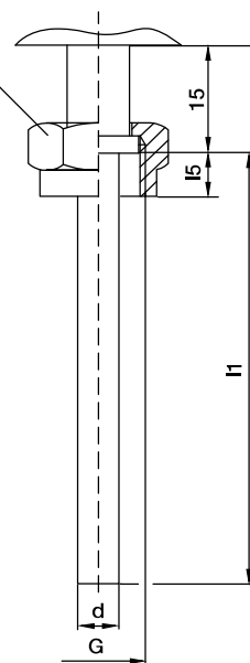
Form 5 Überwurfmutter union nut écrou chapeau
