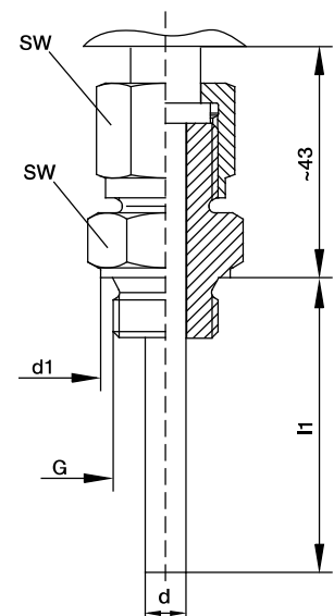
Form 9 Überwurfmutter mit Doppelnippel coupling nut with double nipple écrou avec double mamelle
