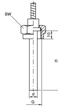
Form 5 Überwurfmutter union nut écrou chapeau
