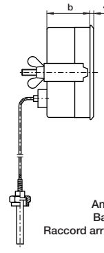
Typ G25.H.2.N... Anschluss hinten mit Rand vorne Back connection with panel mounting flange Raccord arrière, montage par colerette avant
