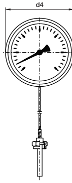
Typ G25.U.3.N... Anschluss unten mit Rand hinten Bottom connection with surface mounting flange Raccord en bas avec montage par rebord arrière
