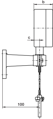
Typ G25.U.1.N... Anschluss unten Bottom connection Raccord en bas
